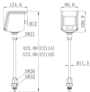
F211x dimension schematic
