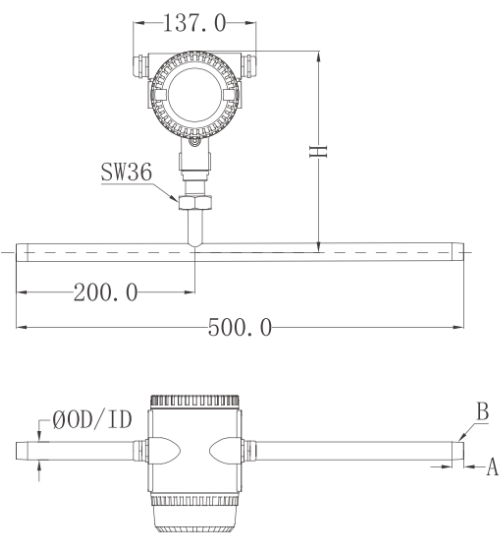
图 3-1 F212x-Ex 螺纹型尺寸示意图
