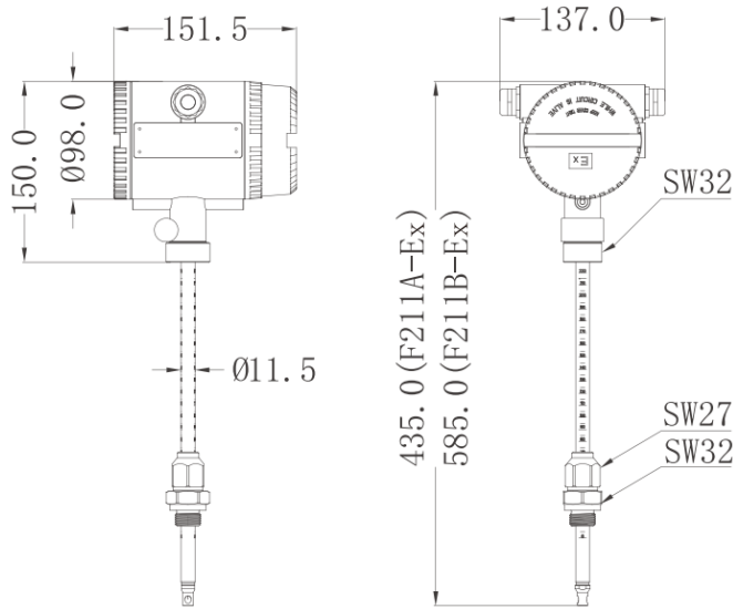
图 3-3 F211x-Ex 尺寸示意图
