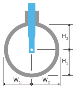
图 3-4 测量点选择示意
