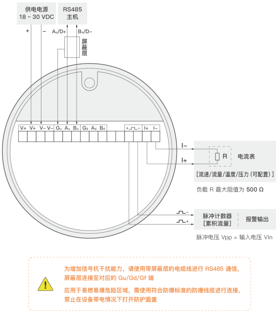
图 3-7 一体式流量计接线示意图
