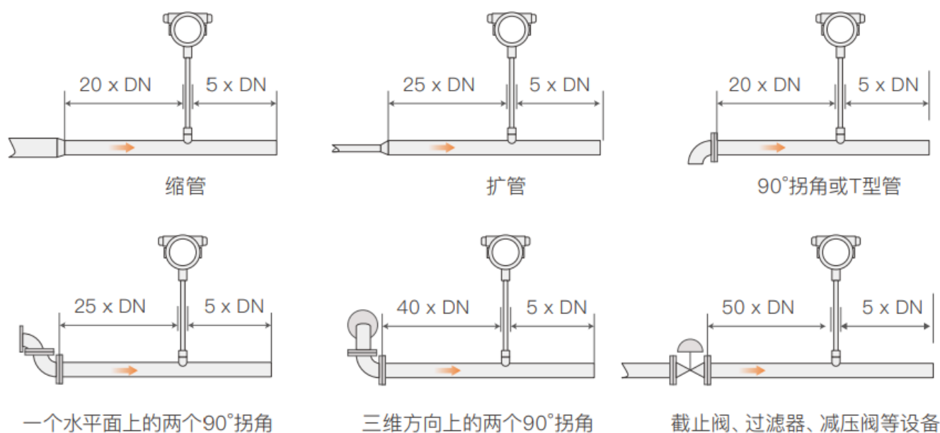
图 3-5 直管段安装要求
