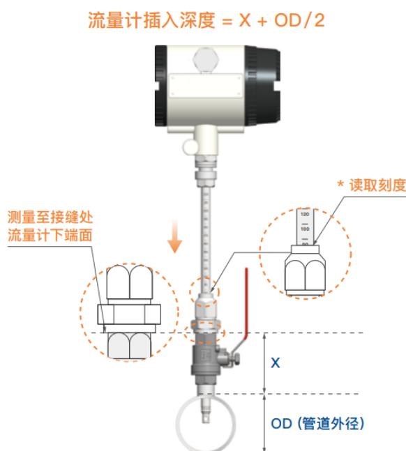
图 3-6 直管段安装要求
