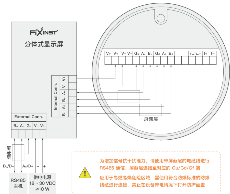
图 3-8 分体式流量计接线示意图
