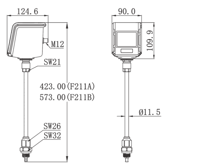
图 3-3 F211x 尺寸示意图
