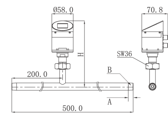
图 3-1 F222x 螺纹型尺寸示意图
