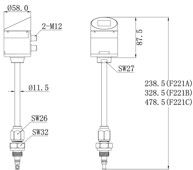
图 3-3 F221x 尺寸示意图
