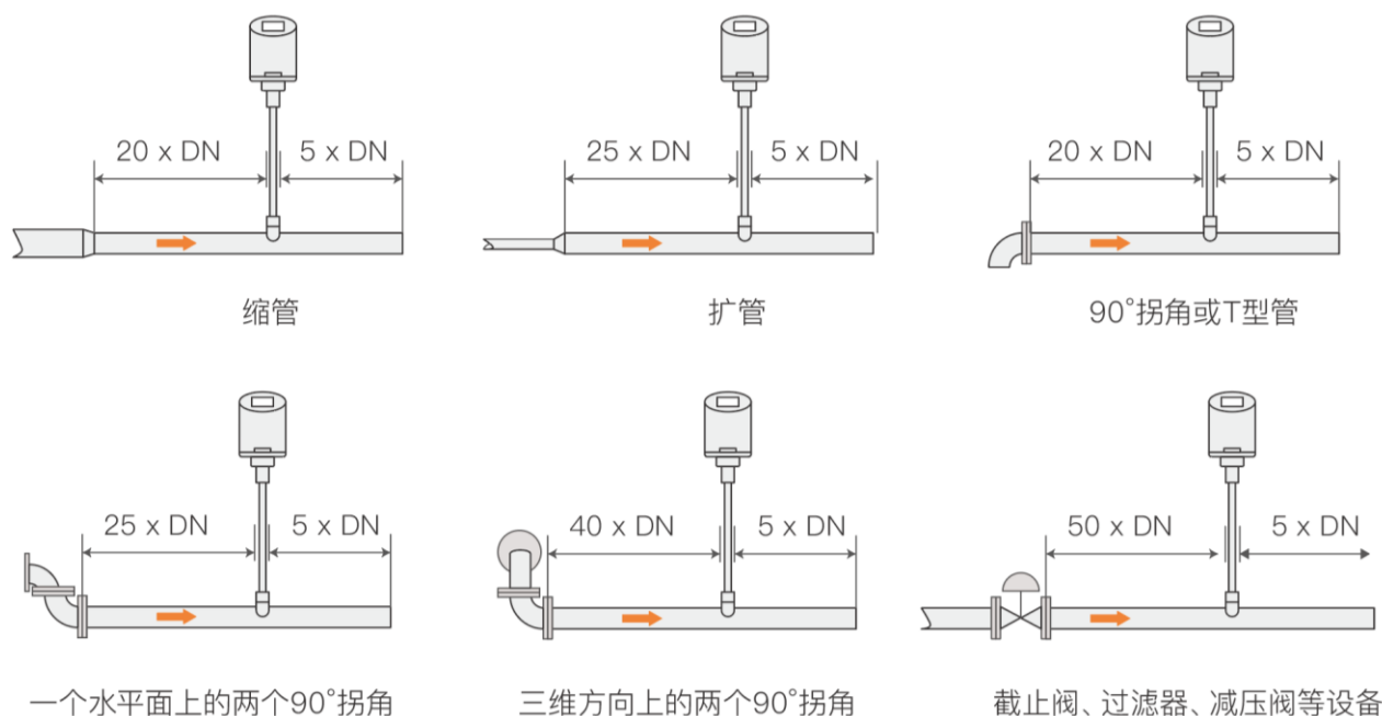
图 3-5 直管段安装要求
