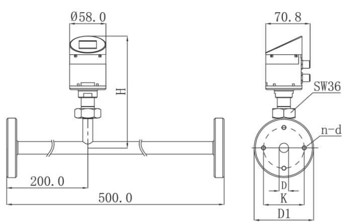
图 3-2 F222x 法兰型尺寸示意图
