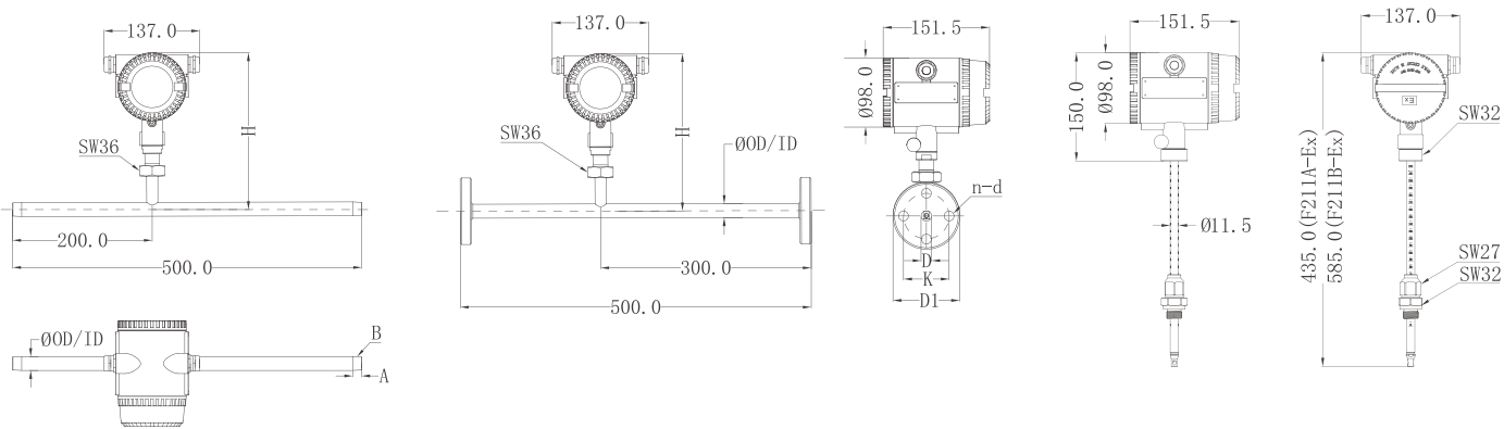
—— F212x-Ex 螺纹型尺寸示意图 —— —— F212x-Ex 法兰型尺寸示意图 —— —— F211x-Ex 尺寸示意图 ——
