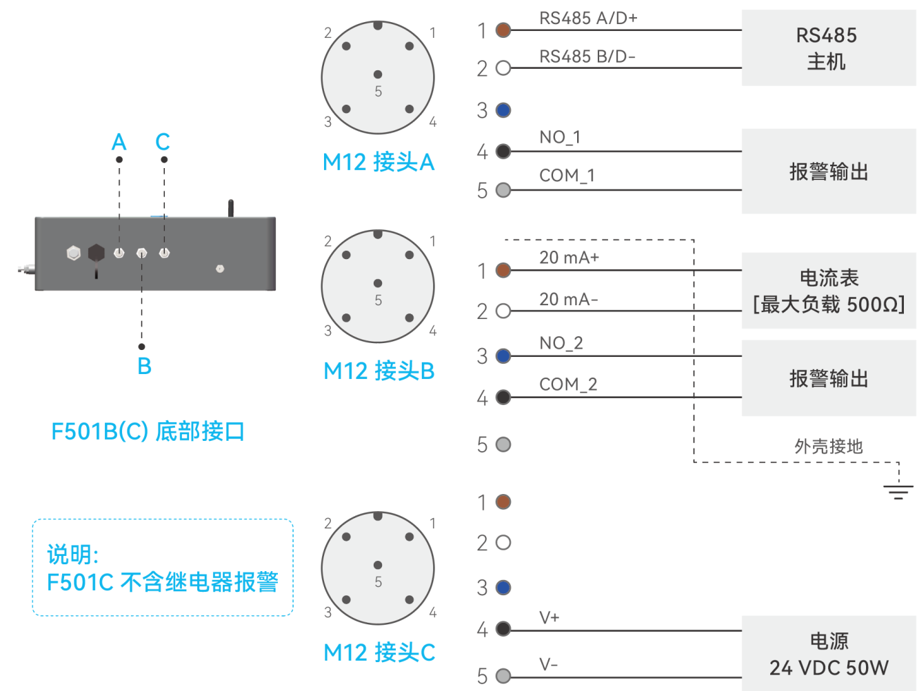
图 3-3 电气接线示意图
