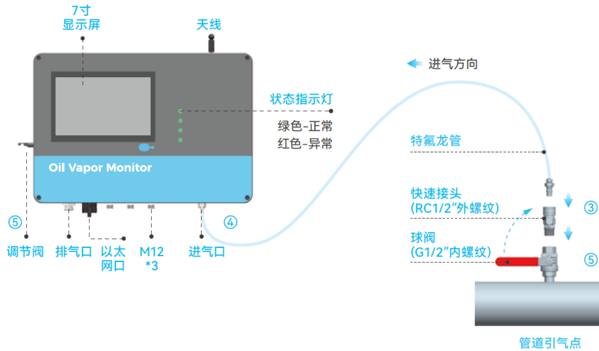
图 3-2 F501B(C) 连接示意
