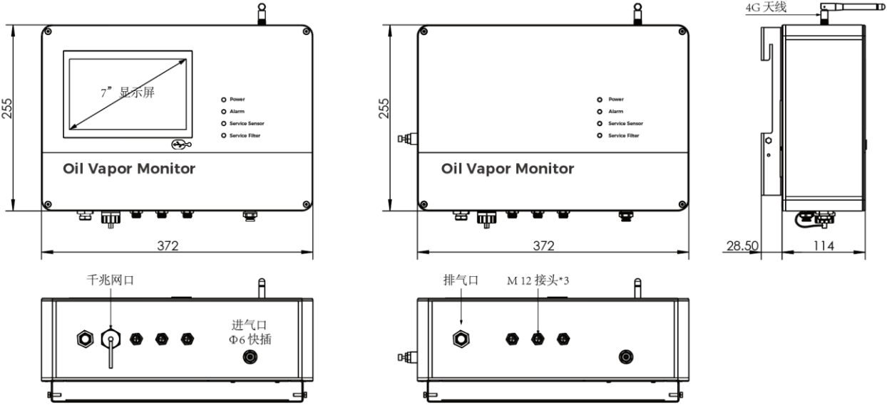
— F501B 产品尺寸 & 功能图 —
